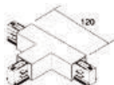
FD765610 Right T joint Правый Т-образный соединитель Figura T derecha
