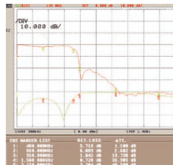
Tap TV A/F response and return loss Tap TV A/F потери на выходе и возвратные Respuesta y pérdidas retorno de la toma TV A/F
